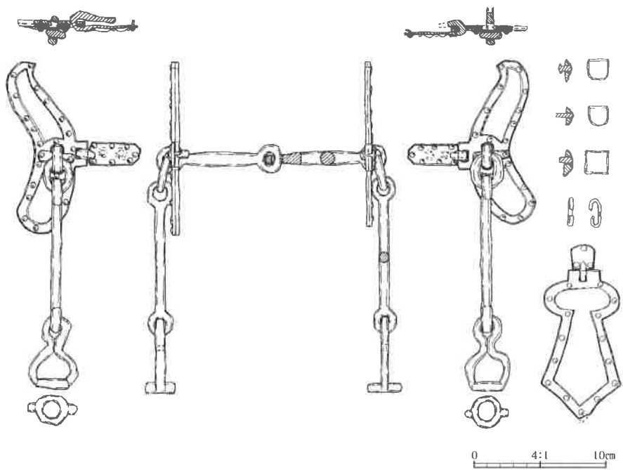
新井原・高岡古墳群4号土壙 馬具 (1988 長野県史刊行会を加筆修正)
