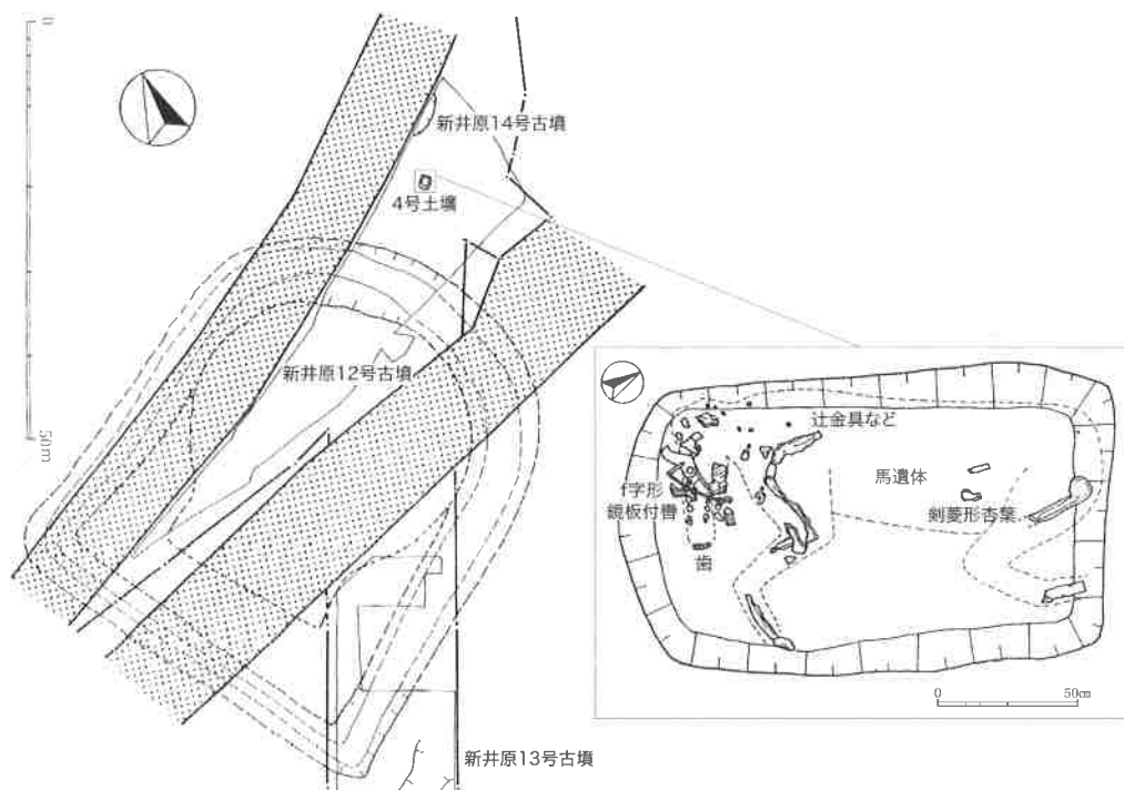
新井原・高岡古墳群4号土壙 馬具・馬遺体出土状況 (1991 下伊那史教育会を加筆修正)
