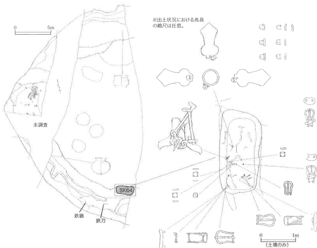
飯田市宮垣外遺跡 SM03(SK64) 遺物・馬骨出土状況 (小林・澁谷 2000を加筆修正)
