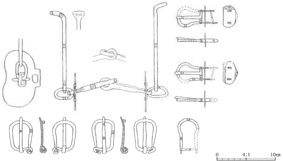
千葉県佐倉市 大作31号墳1号 土墳出土馬具(1990 藤崎・田島を加筆修正) 一周溝を掘り込む事例—①
