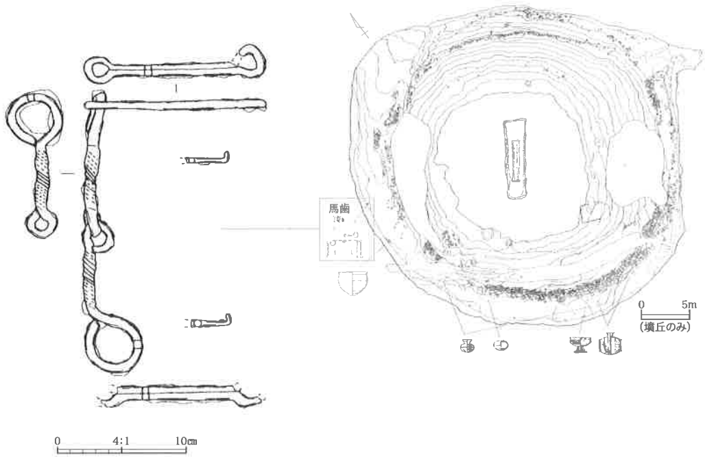
飯田市 物見塚古墳 轡・馬齒(小林 1992を加筆修正)
