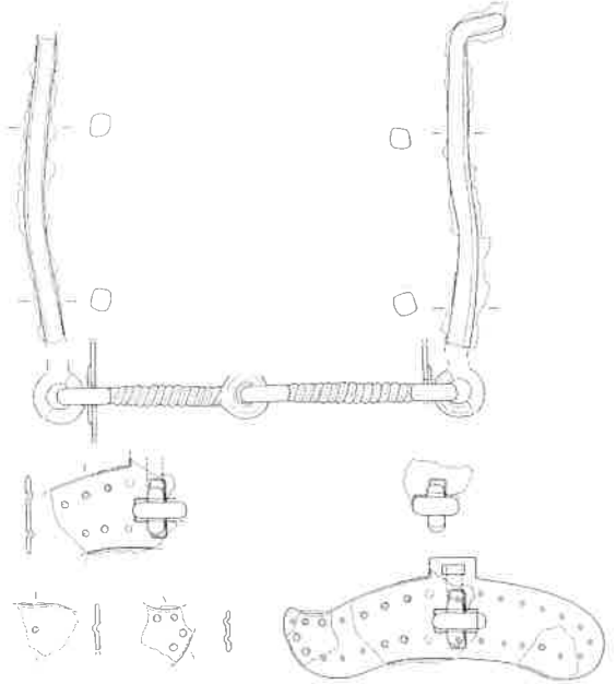
福井県松岡町(永平寺町) 鳥越山古墳 (松岡町教育委員会・永平寺町教育委員会 2005を加筆修正) ※鏡板の復元は筆者作成。
